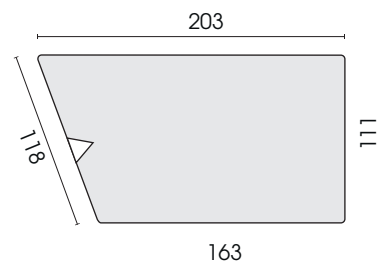
Segment 2-Sitz rechts 215t
