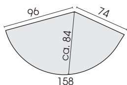
Hocker, halbrund, links 530L
